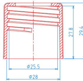
(30/400) CAP, P=1"x8 TPI
