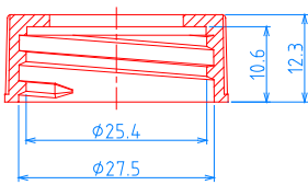
(28/400) CAP, P=1"x8 TPI
