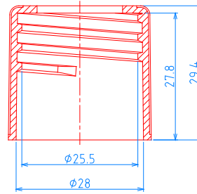
(30/400) CAP, P=1"x8 TPI
