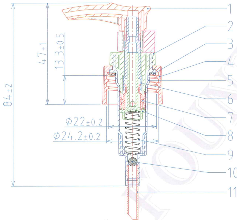
(24/410) CAP, P=1"x8 TPI
