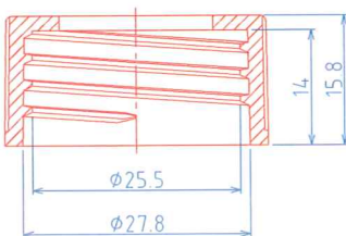
(28/400) CAP, P=1"x8 TPI
