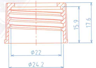
(24/415) CAP, P=1"x8 TPI
