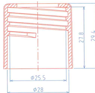
(30/400) CAP, P=1"x8 TPI
