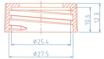
(28/400) CAP, P=1"x8 TPI
