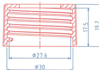
(30/400) CAP, P=1"x8 TPI
