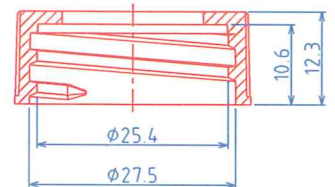
(28/400) CAP, P=1"x8 TPI
