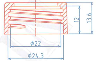
(24/410) CAP, P=1"x8 TPI
