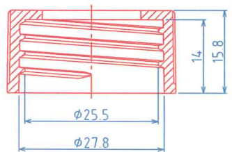
(28/400) CAP, P=1"x8 TPI
