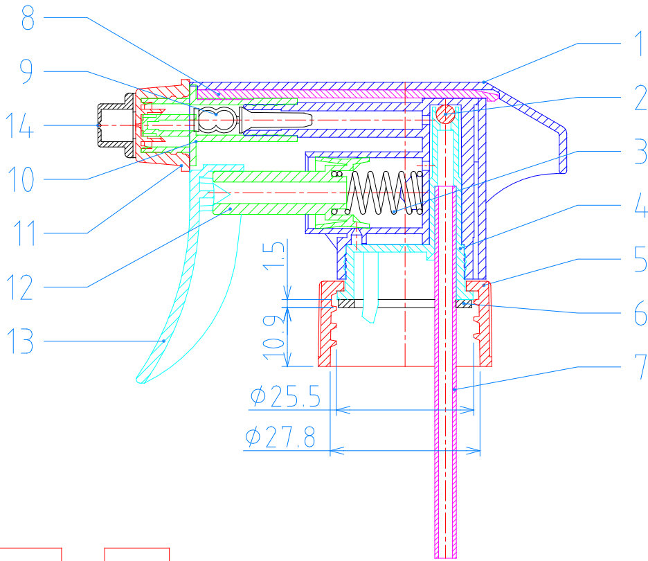
(28/400W) CAP , P=1"x8 TPI
